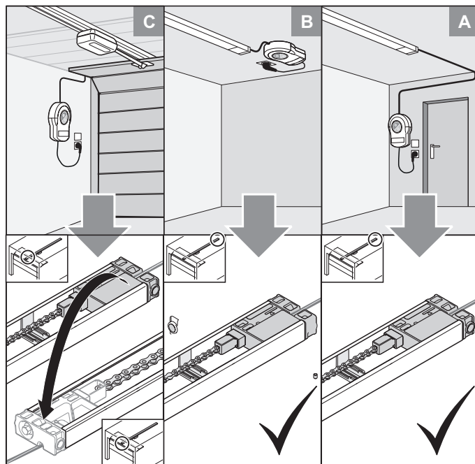
Ábra: A, B és C beszerelési helyzet
