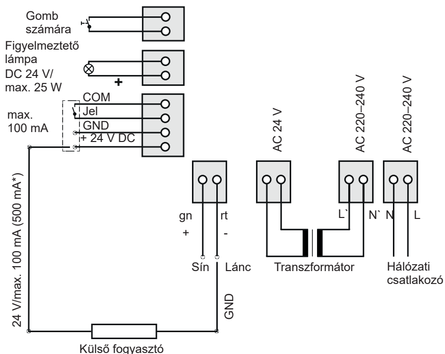
Ábra. Fali vezérlés bekötési rajz
