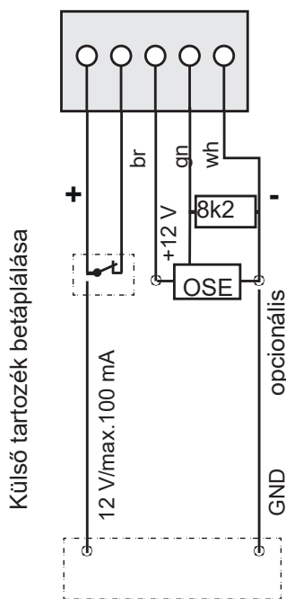
Ábra: Futókocsi bekötési rajz
