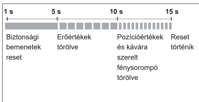
Ábra: A futókocsin lévő állapot LED időfolyamatának áttekintése a zöld reset-gomb megnyomása esetén
