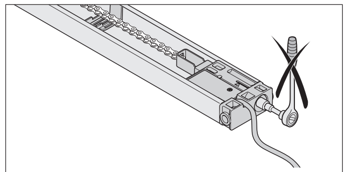
Ábra: Betoló darab vezérlővezetékekkel
